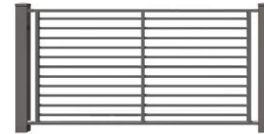
GERADES ZAUNFELD (TYP P) Maximal verfügbare Breite: 3000 mm Minimale Standardbreite: 2000 mm
