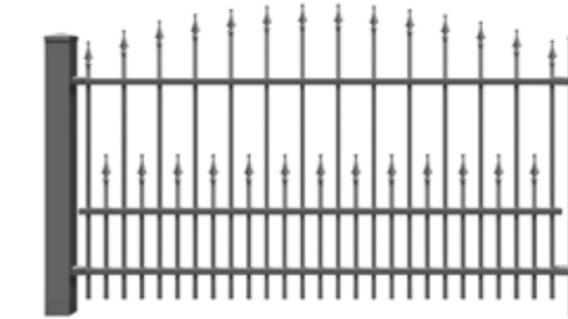
ZAUNFELD MIT BOGEN (TYP W) Maximal verfügbare Breite: 3000 mm Minimale Standardbreite: 2000 mm
