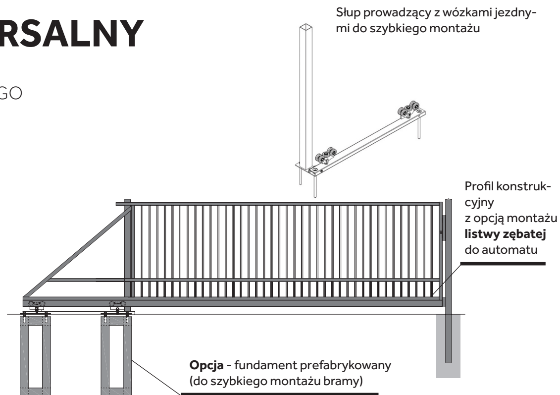
Brama przesuwna
